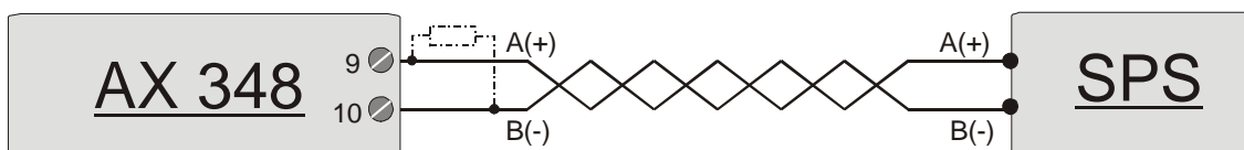
Anschluss der RS485-Schnittstelle
